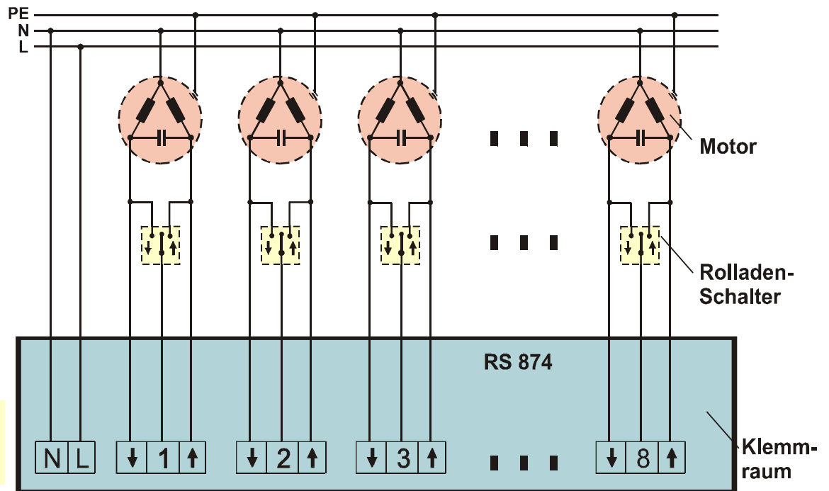
Anschluss- bild (Fig. 1)
