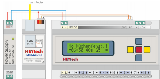
LAN-Modul, M-Serie
