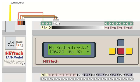
LAN-Modul, L-Serie
